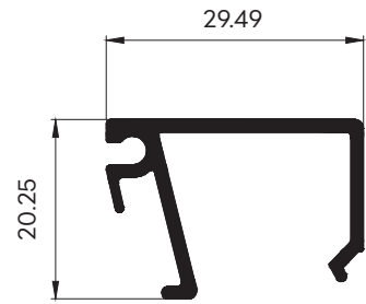
30055 ( GL 6 mm.) WT : 0.315 Kg./m. ตัวบานเปิดร่อง 12.7 มม.
