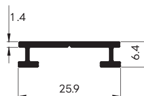
42794 WT : 0.155 Kg./m. ตัวรอง CONNECTING ROD
