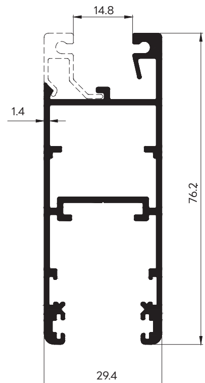
42969 WT : 1.050 Kg./m. กรอบบาน 3 นิ้ว คิ้วปิด
