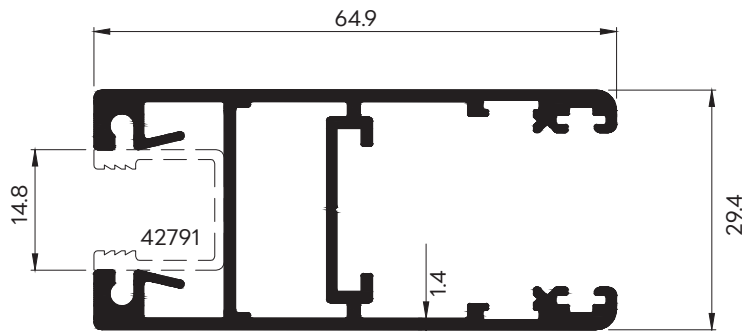
42026 WT : 1.044 Kg./m. กรอบบานร่อน 14.8 มม.
