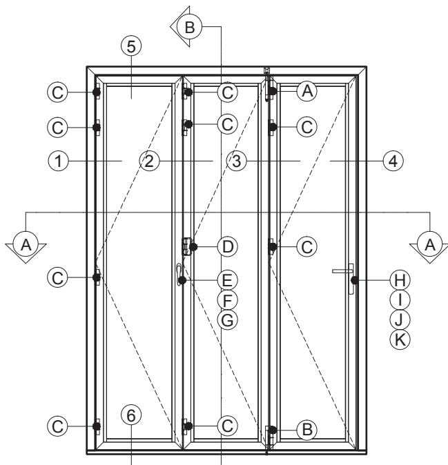
Bottom Pivot Hinge System ล๊อบล่างบานพับ
