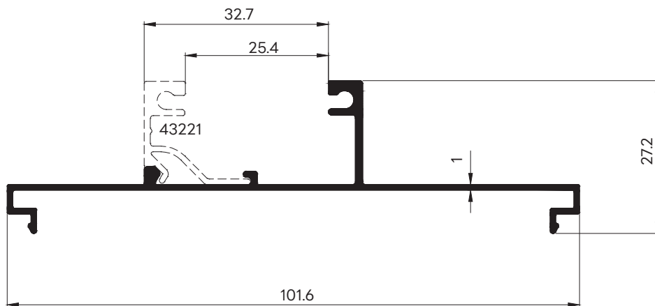
50729 WT : 0.484 Kg./m. ວັດໜັກສ່ວນ (101.6 มม.)
