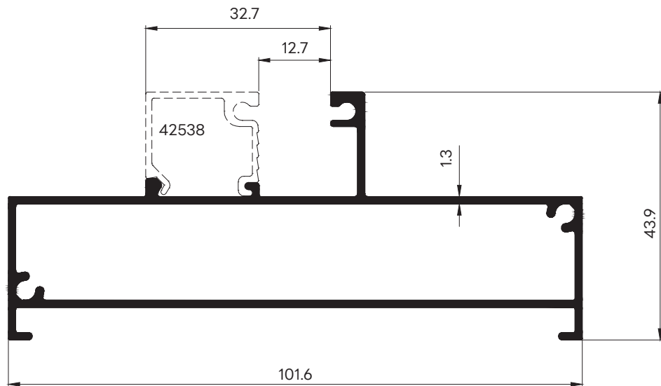
50728 WT : 1.081 Kg./m. ວັດໜັກສ່ວນ (101.6 มม.)
