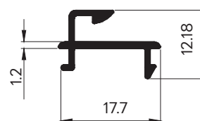
20007 WT : 0.131 Kg./m. เสริมมุมอลูมิเนียม
