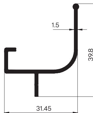
42109 WT : 0.322 Kg./m. ກະທຸກຄຸນນ້ຳ
