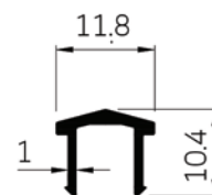
42310 WT : 0.090 Kg./m.
