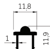
42311 WT : 0.125 Kg./m.
