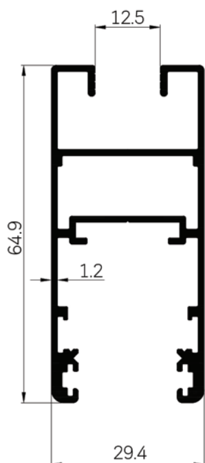
43068 WT : 0.886 Kg./m.
