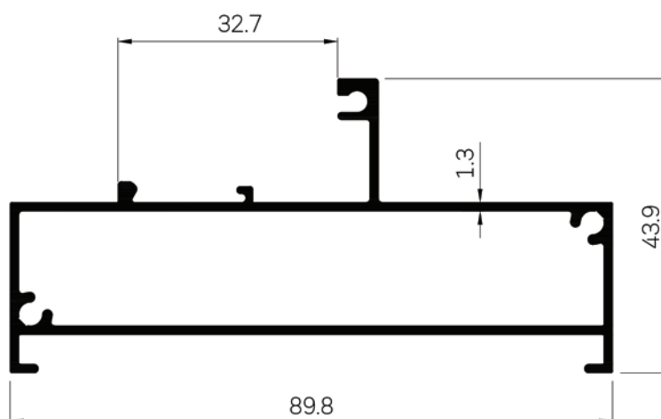
42559 WT : 0.998 Kg./m.
