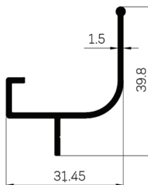
42109 WT : 0.322 Kg./m.
