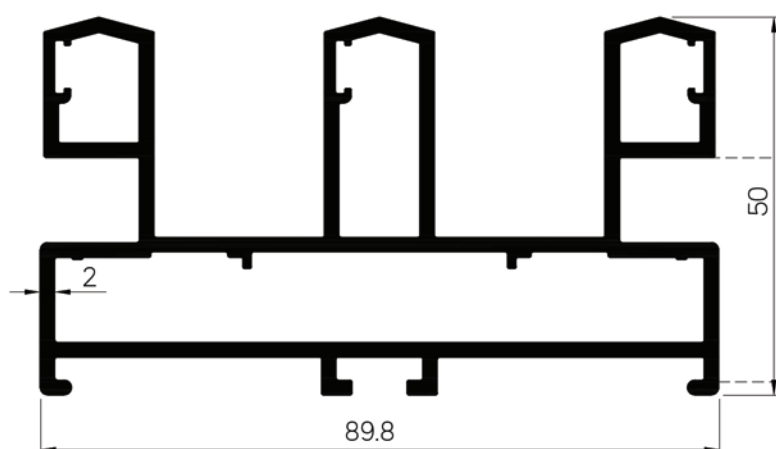
42836 WT : 2.343 Kg./m.
