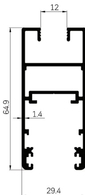
42793 WT : 0.967 Kg./m.
