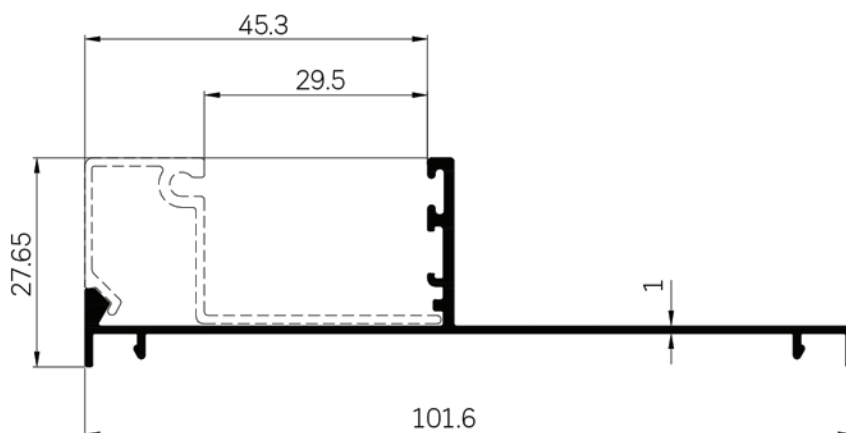
30357 WT : 0.472 Kg./m.
