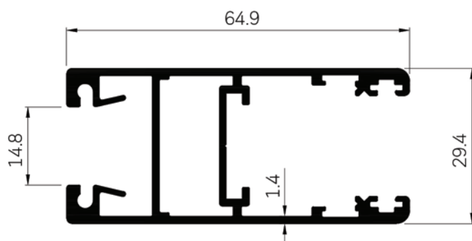
42026 WT : 1.044 Kg./m.
