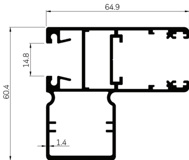
42027 WT : 1.479 Kg./m.
