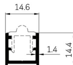
43159 WT : 0.156 Kg./m.
