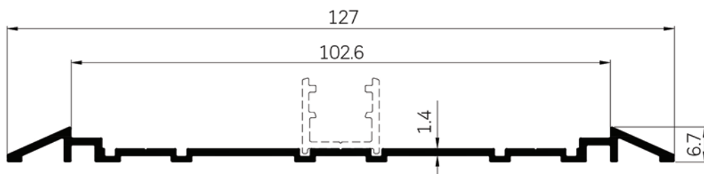
43158 WT : 0.584 Kg./m.
