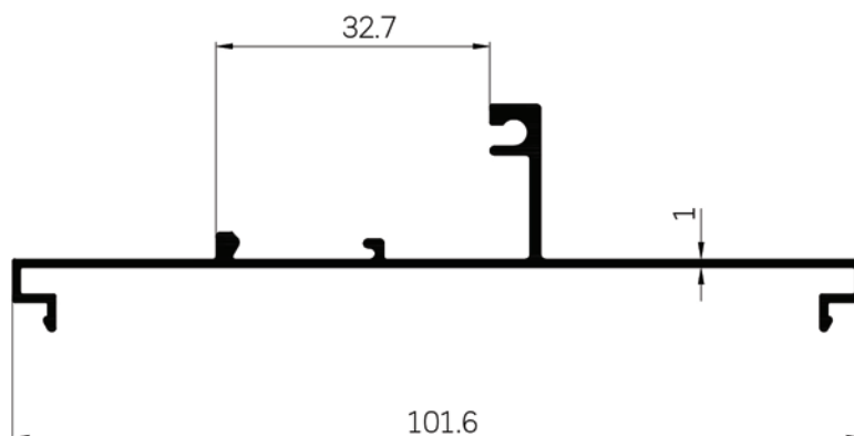
50729 WT : 0.484 Kg./m.
