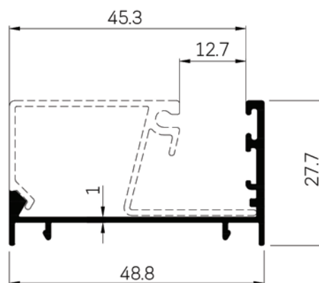
50611 WT : 0.329 Kg./m.
