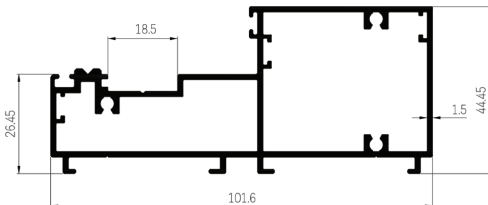
30355 WT : 1.596 Kg./m.
