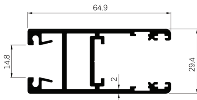
42835 WT : 1.247 Kg./m.
