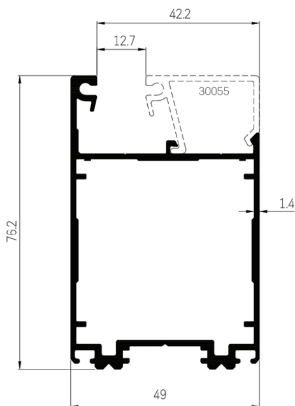
30264 WT : 1.242 Kg./m.
