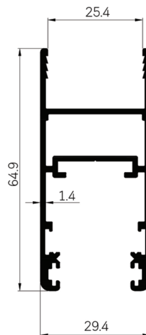
42663 WT : 0.904 Kg./m.
