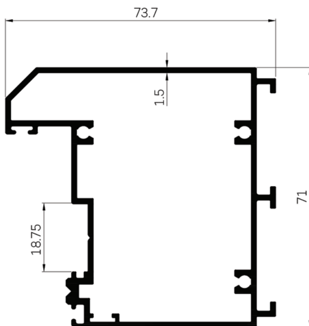
30263 WT : 1.459 Kg./m.
