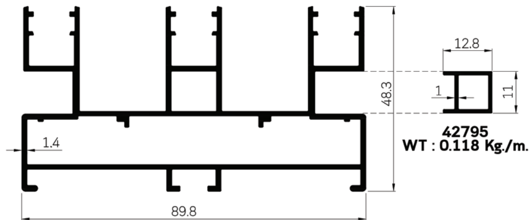
42788 WT : 0.202 Kg/m.
