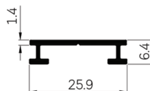
42794 WT : 0.155 Kg./m.
