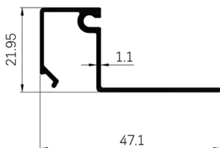
50726 WT : 0.292 Kg./m.
