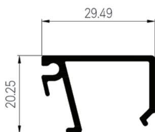
30055 WT : 0.315 Kg./m.
