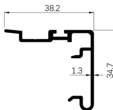
42028 WT : 0.382 Kg./m.
