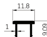
42792 WT : 0.093 Kg./m.
