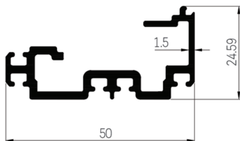
30061 WT : 0.678 Kg./m.
