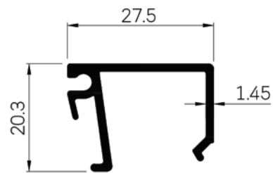
30056 WT : 0.304 Kg./m.
