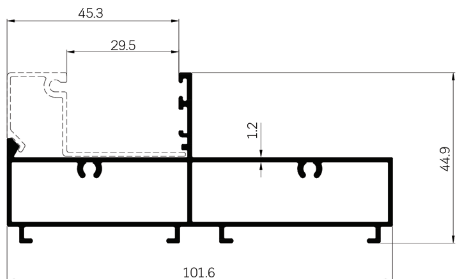
30356 WT : 1.118 Kg./m.
