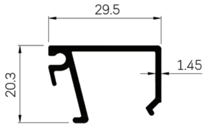
30055 WT : 0.315 Kg./m.
