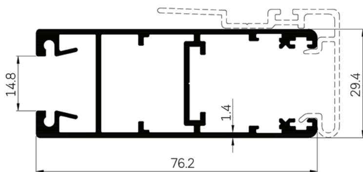
42664 WT : 1.157 Kg./m.
