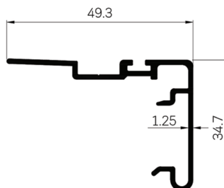
42665 WT : 0.422 Kg./m.
