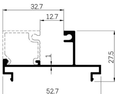
42539 WT : 0.349 Kg./m.
