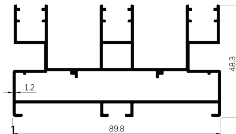
43067 WT : 1.462 Kg./m.
