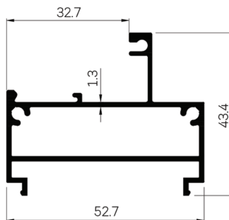
42537 WT : 0.737 Kg./m.
