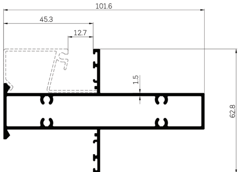
30252 WT : 1.398 Kg./m.
