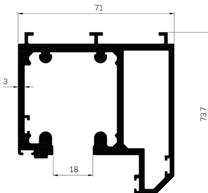
30063 WT : 2.961 Kg./m.
