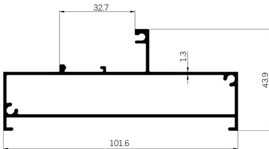
50728 WT : 1.081 Kg./m.
