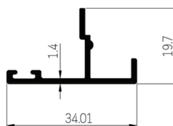
30066 WT : 0.246 Kg./m.
