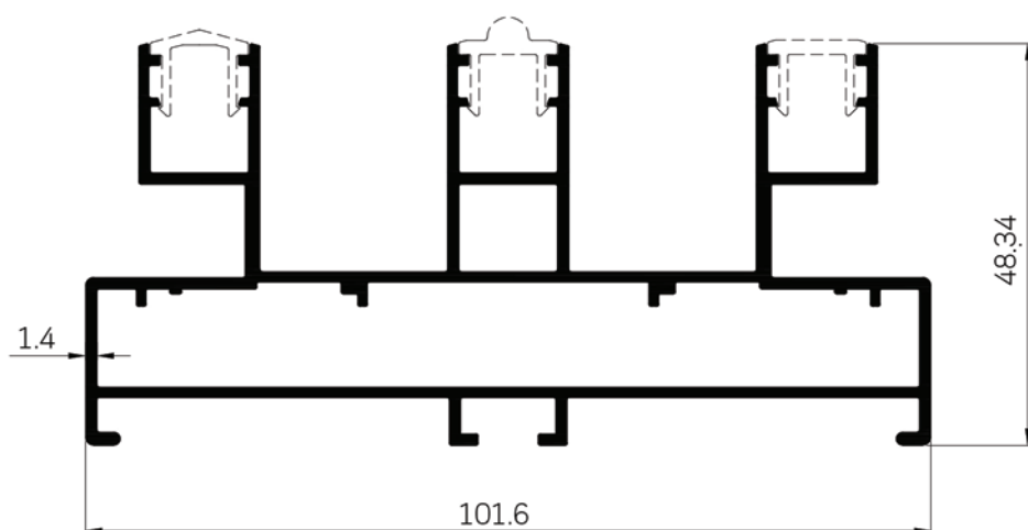
42787 WT : 1.701 Kg./m.
