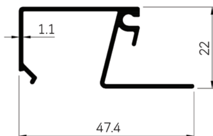
50612 WT : 0.350 Kg./m.
