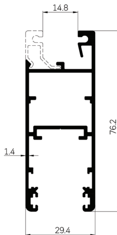
42969 WT : 1.050 Kg./m.
