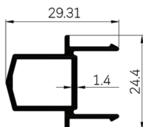
42042 WT : 0.318 Kg./m.
