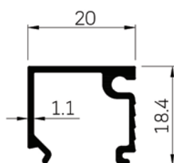
42538 WT : 0.207 Kg./m.
