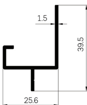
42562 WT : 0.308 Kg./m.
