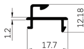
20007 WT : 0.131 Kg./m.
