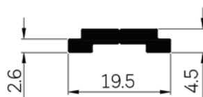
42029 WT : 0.167 Kg./m.
