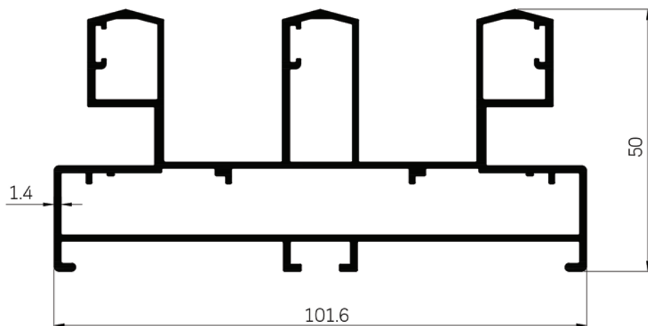
42778 WT : 1.783 Kg./m.
