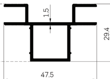
42111 WT : 0.574 Kg./m.
