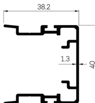
42446 WT : 0.573 Kg./m.
