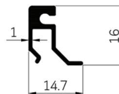
42970 WT : 0.159 Kg./m.
