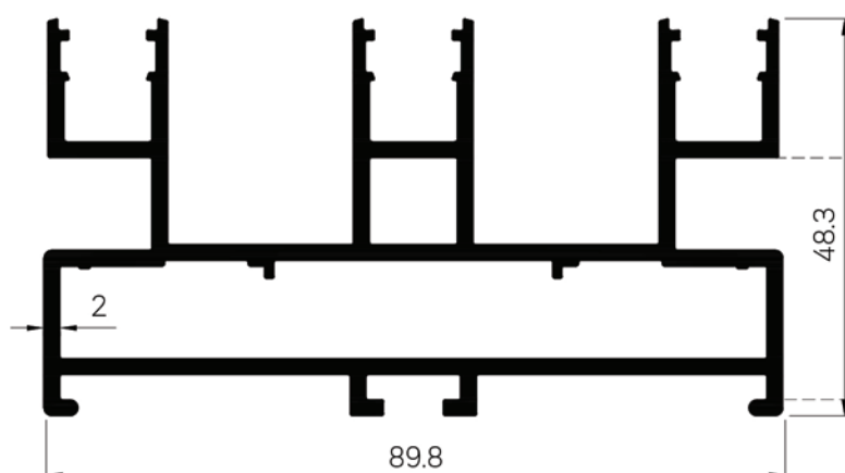
42837 WT : 2.197 Kg./m.
