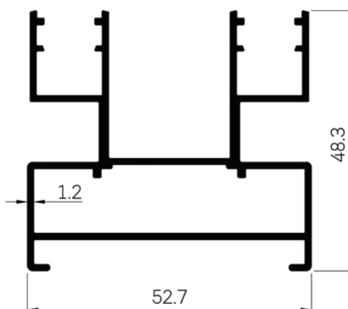
43066 WT : 0.930 Kg./m.
