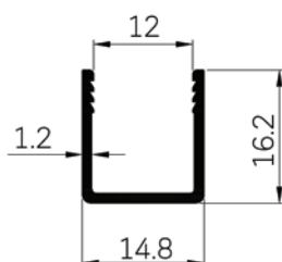
42790 WT : 0.146 Kg./m.
