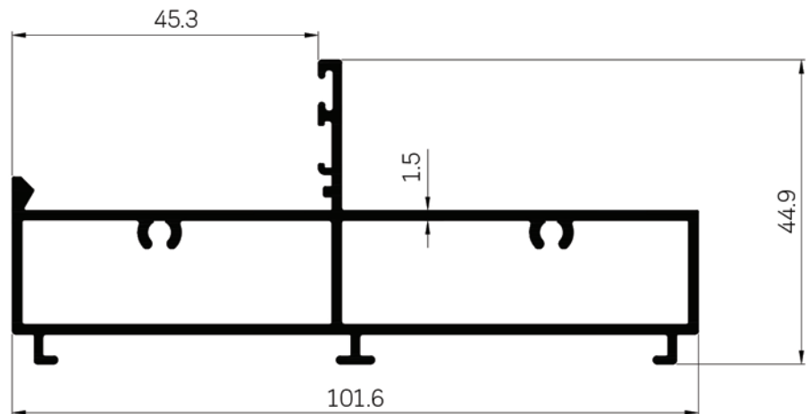
30250 WT : 1.306 Kg./m.
